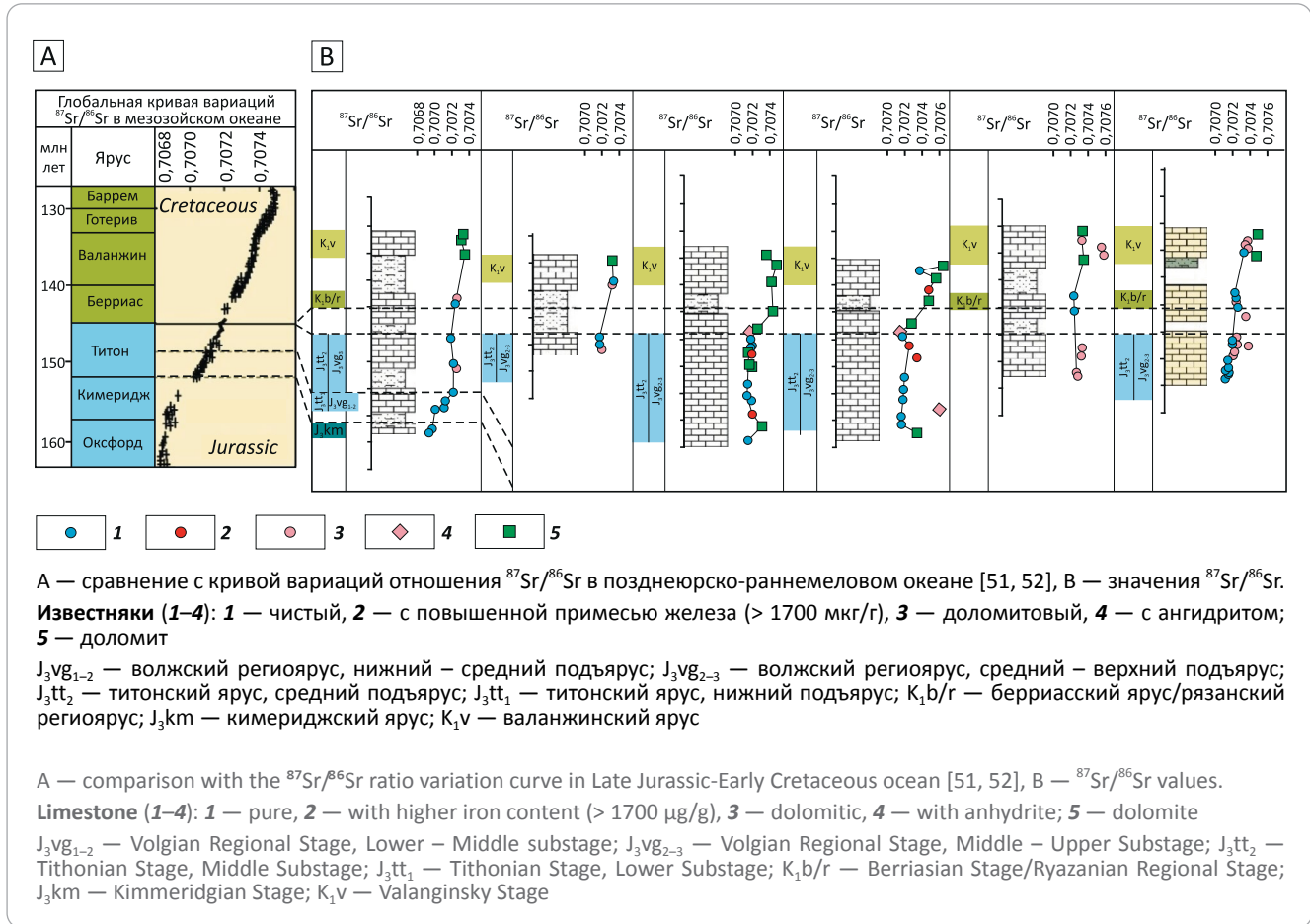
Рис. 8. Фрагмент схемы корреляция карбонатных пород изученных скважин на основе значений ^{87}\text{Sr}/^{86}\text{Sr} Fig. 8. Fragment of the correlation chart for carbonate rocks in the studied wells based on ^{87}\text{Sr}/^{86}\text{Sr} values
