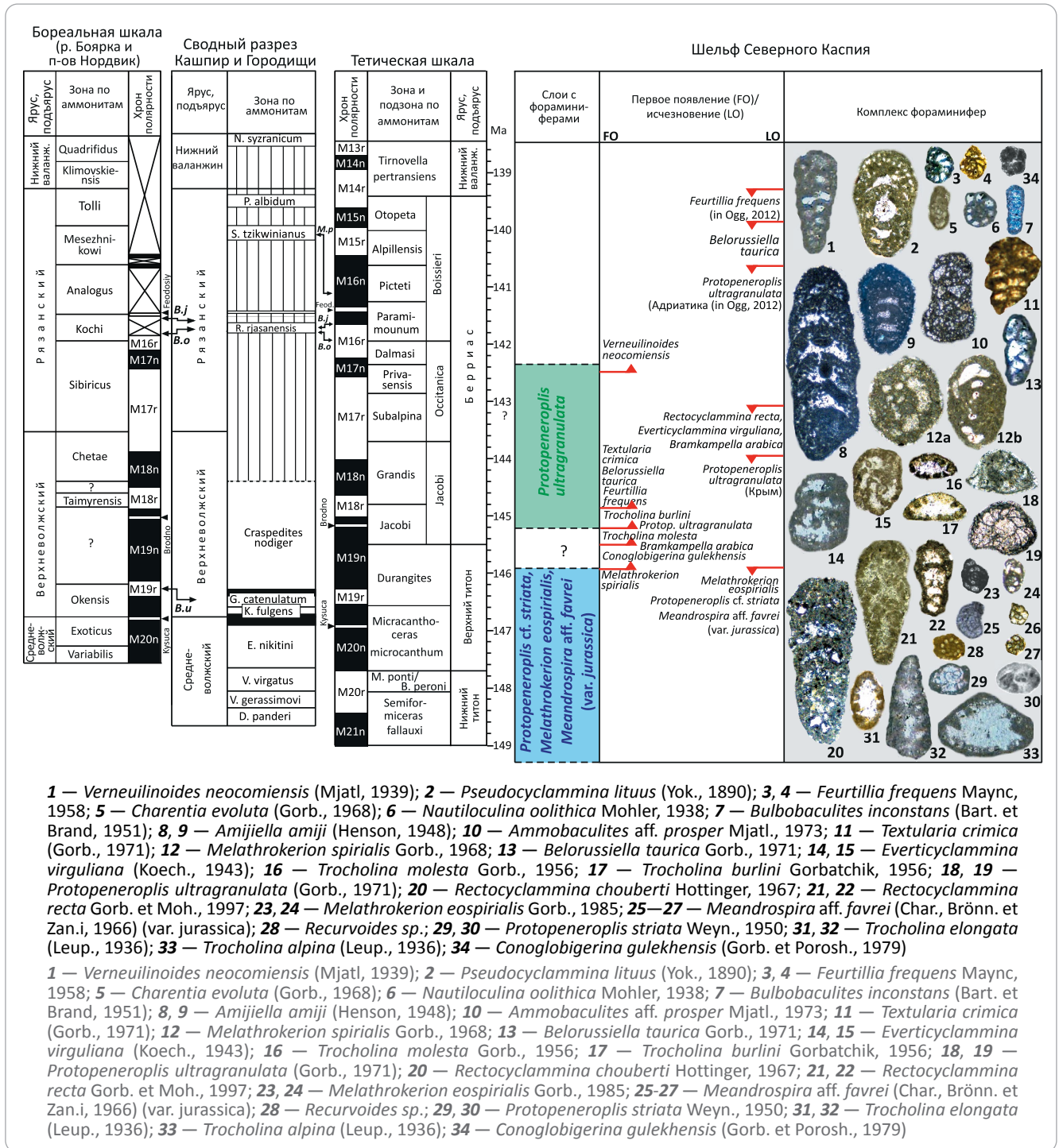
Рис. 3. Фораминиферы титон-берриасских отложений северной части шельфа Каспийского моря (по [4, 9]) Fig. 3. Foraminifera of the Tithonian-Berriasian deposits in the northern part of the Caspian shelf [4, 9]
